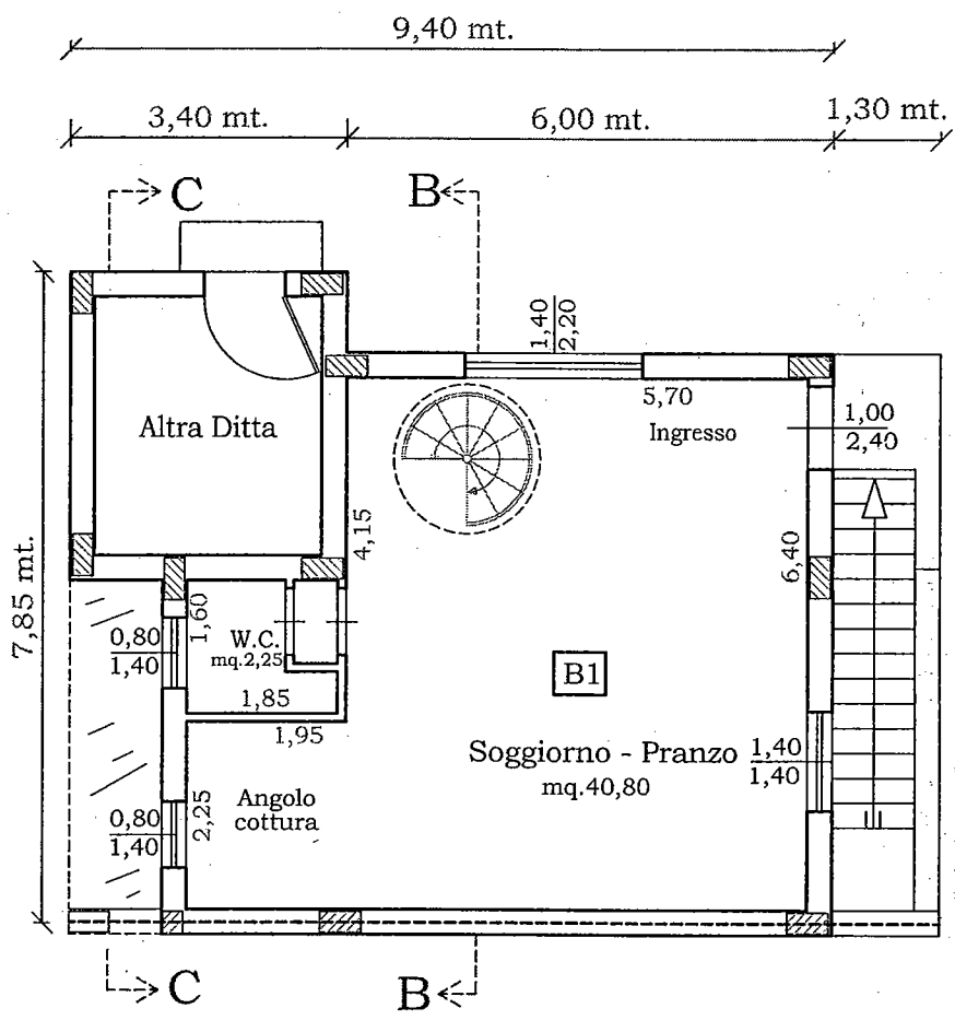
Pianta Piano Terreno Disegno Scala 1:100 Unità Immobiliare "B1"
