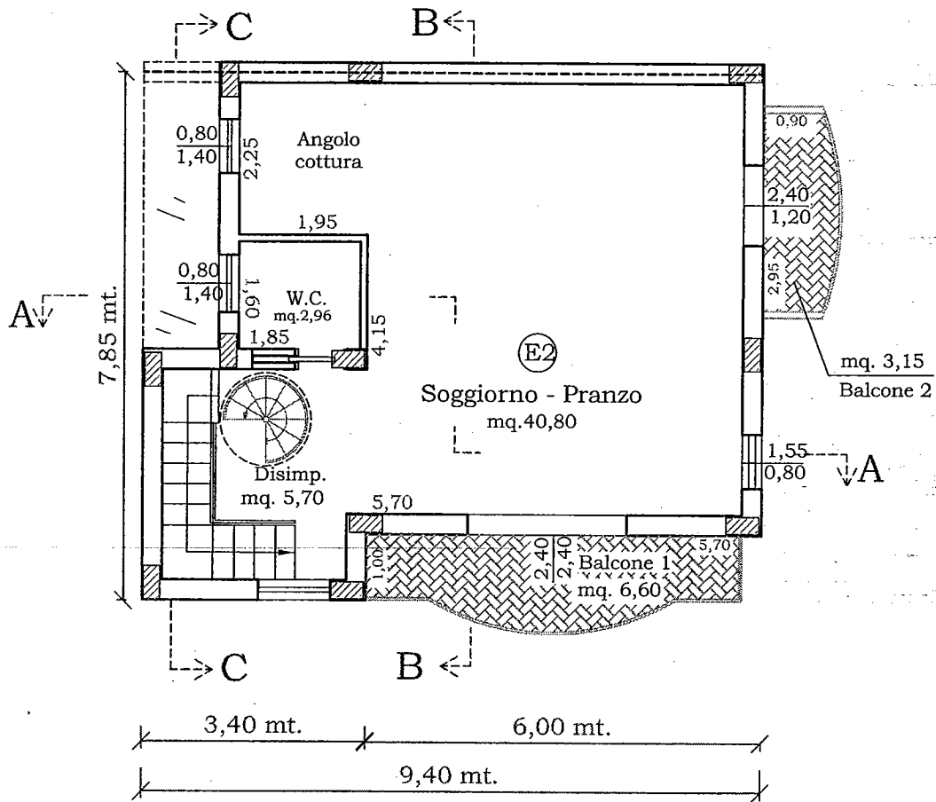
Pianta Piano Primo Disegno Scala 1:100 Unità Immobiliare "E2"
