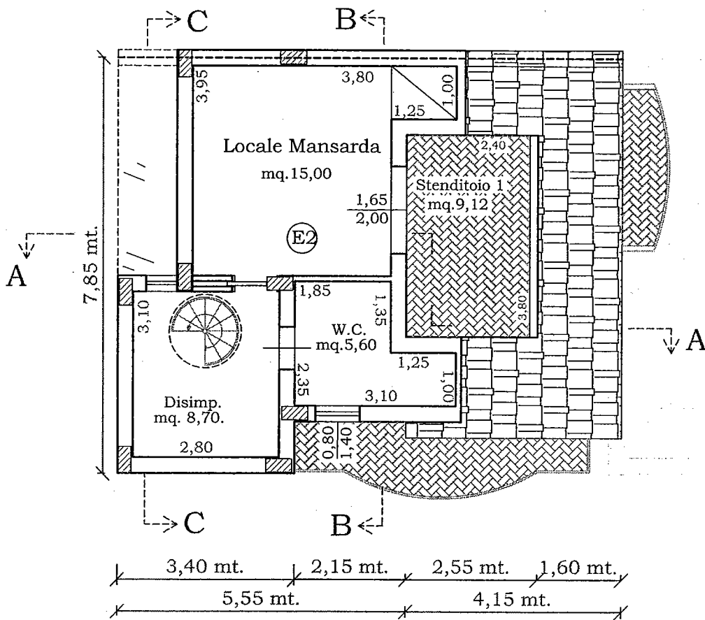
Pianta Piano Sottotetto Disegno Scala 1:100 Unità Immobiliare "E2"
