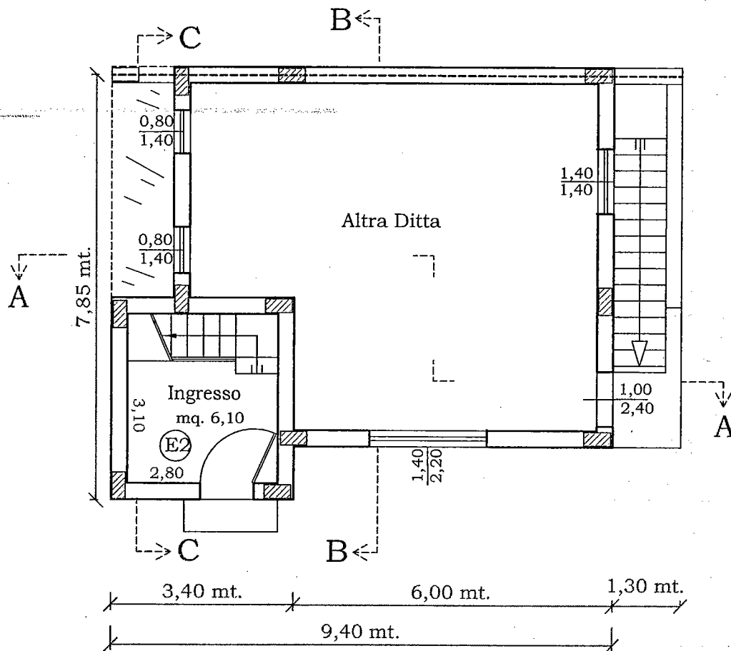
Pianta Piano Terreno Disegno Scala 1:100 Unità Immobiliare "E2"
