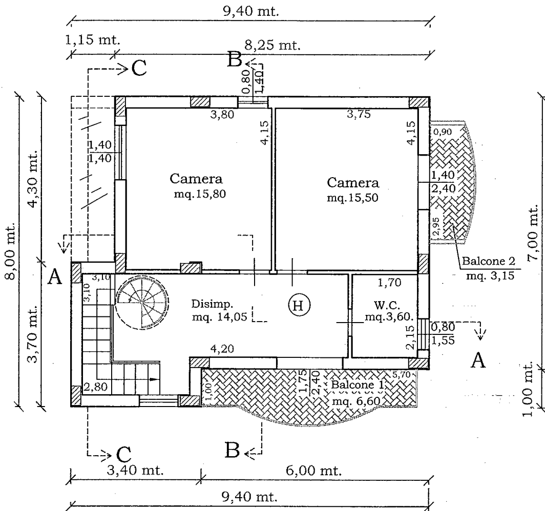
Pianta Piano Primo Disegno Scala 1:100 Unità Immobiliare "H"
