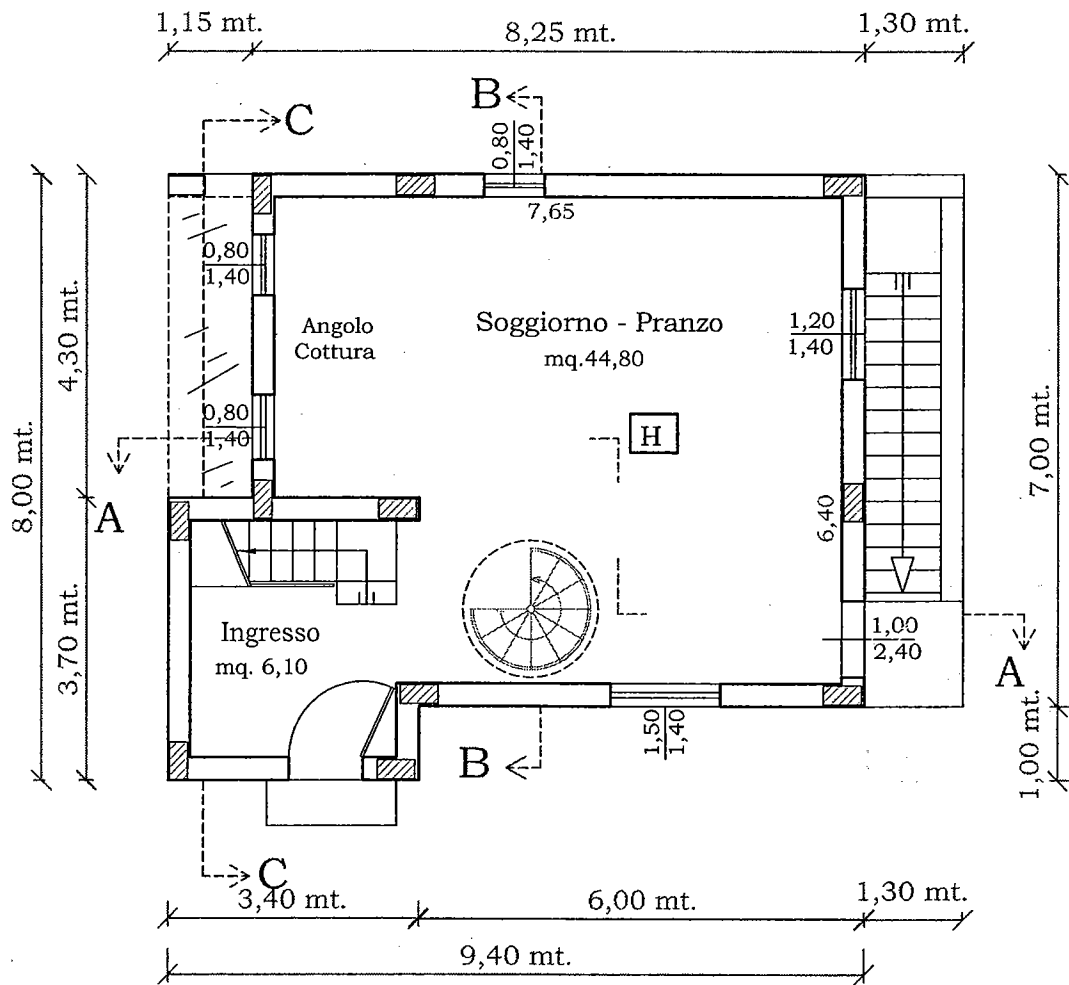
Pianta Piano Terreno Disegno Scala 1:100 Unità Immobiliare "H"
